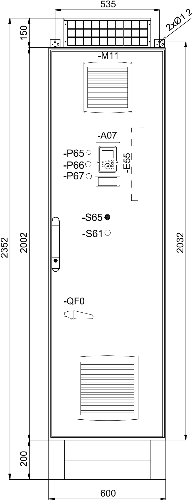
Prednji pogled
